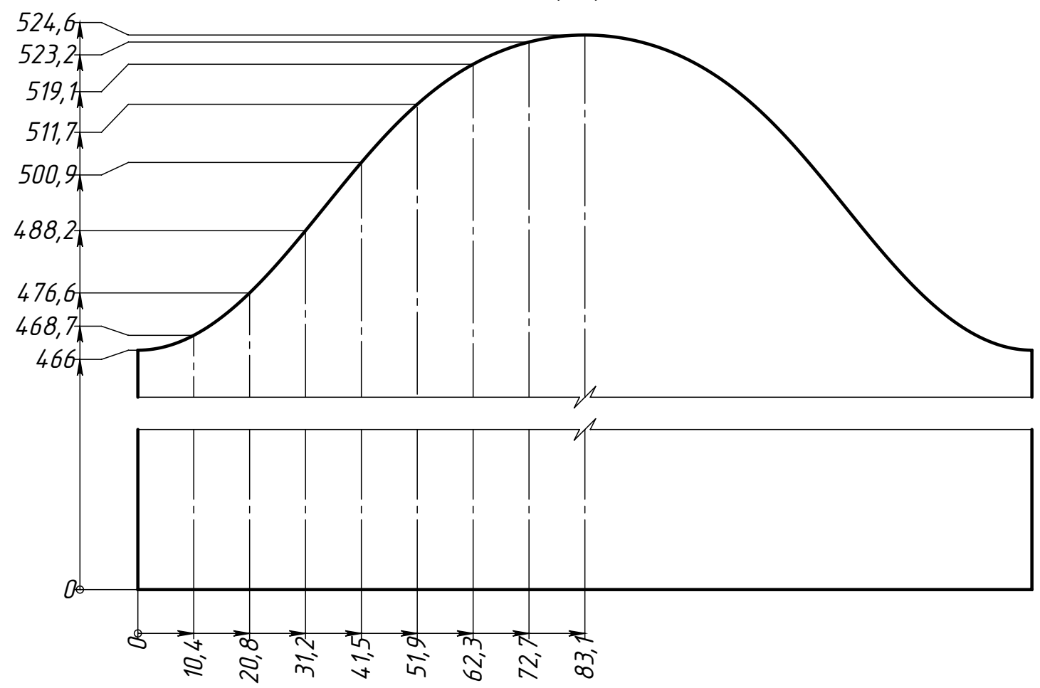
Поз.4 (Стойка) Развертка 1 : 1
